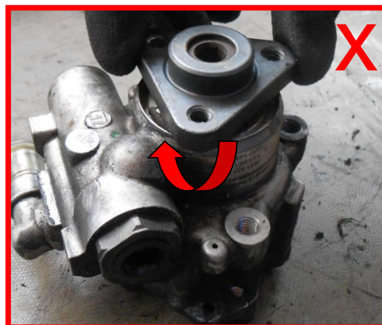
Welle schwergängig / nicht drehbar → unzulässig
